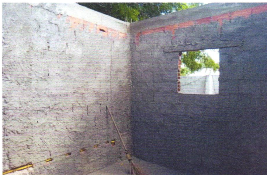
FOTO 07 - CHAPISCO APLICADO EM ALVENARIA (COM PRESENÇA DE VÃOS) E ESTRUTURAS DE CONCRETO DE FACHADA, COM COLHER DE PEDREIRO. ARGAMASSA TRAÇO 1:3 COM PREPARO EM BETONEIRA 400L. AF_10/2022
