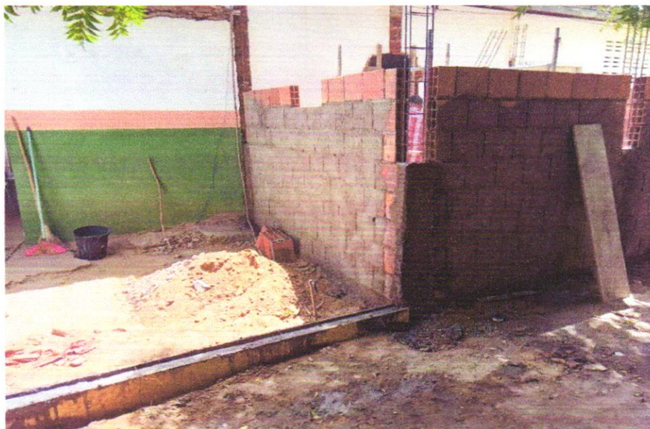
FOTO 05 - Alvenaria bloco cerâmico vedação, 9x19x24cm, e=9cm, com argamassa t5 - 1:2:8 (cimento/cal/areia), junta=1cm - Rev.09
